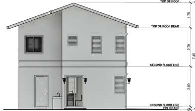
5 LEFT SIDE ELEVATION A-1 1:75
